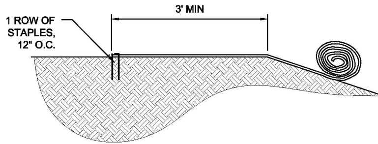
TOP OF SLOPE ANCHOR EXAMPLE 1 N.T.S.
